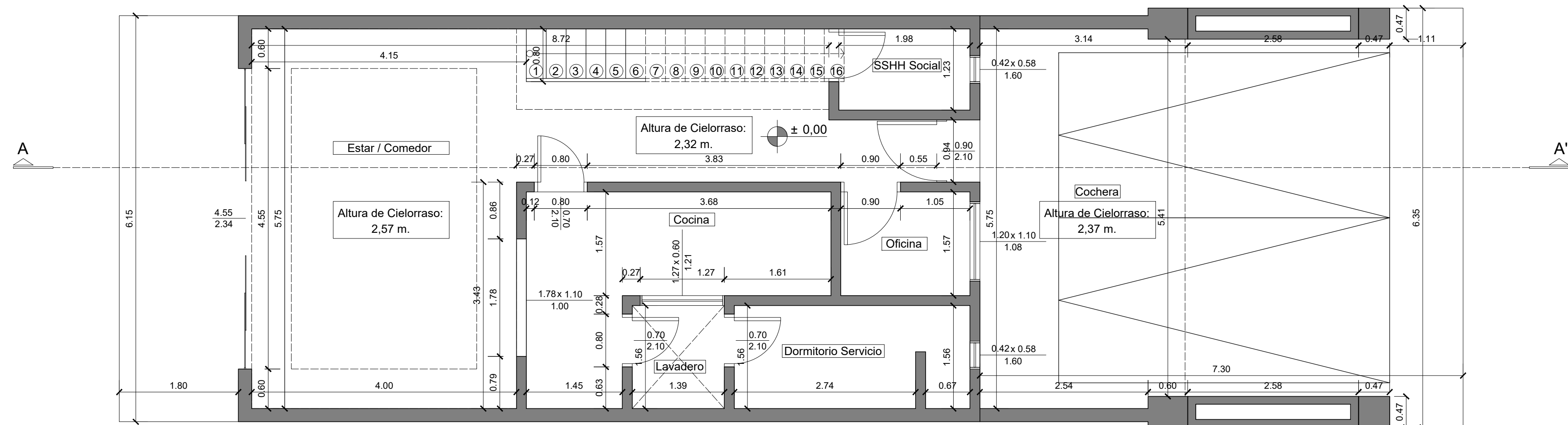
Planta Baja
