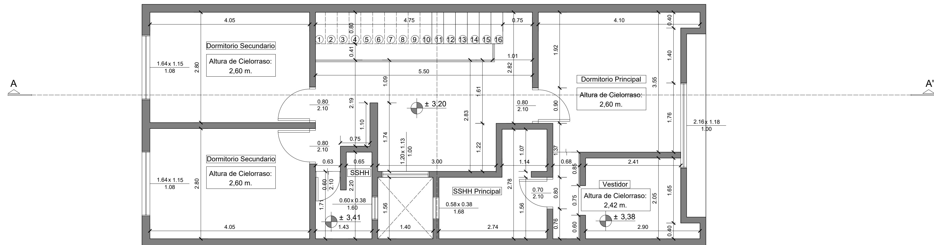
Planta Alta
